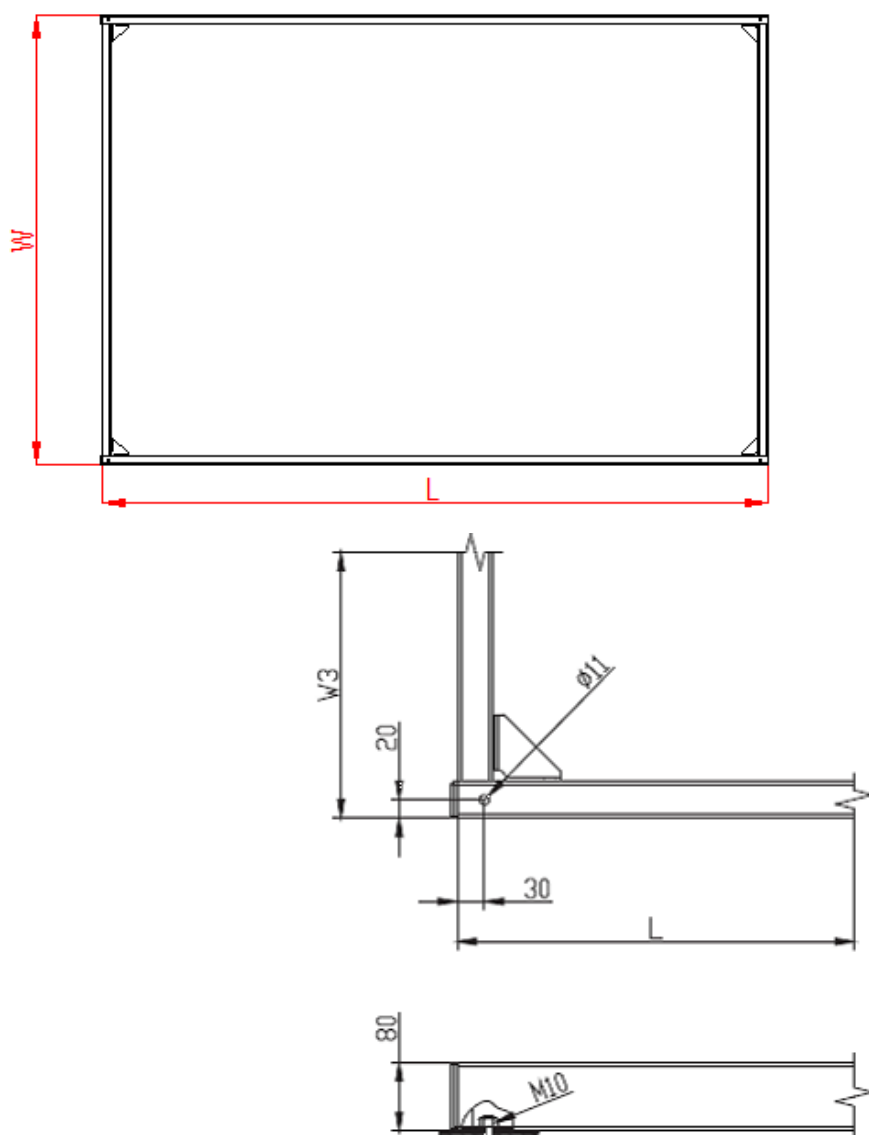
Rys.12d Usytuowanie skrajnych otworów fundamentowych i przykład kotwienia central VS 21-650
