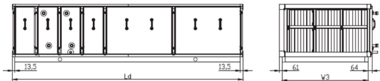
Rys.12b. Ramy transportowe z profilu zamkniętego o przekroju prostokątnym central VS 21-650
